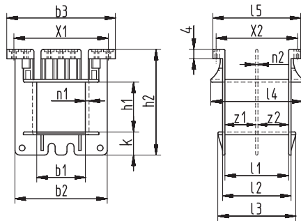
Schemazeichnung | Schematic drawing
