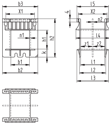
Schemazeichnung | Schematic drawing
